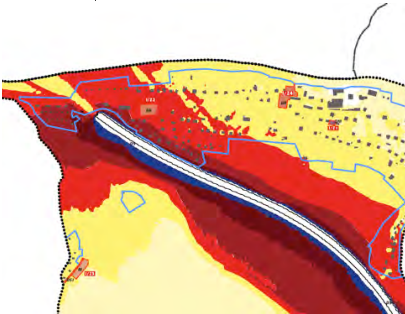
hodnoty hladiny hlukového ukazatele L_{dvn} strategických hlukových map silnic ČR z r. 2017 a vyznačení lokalit změn
